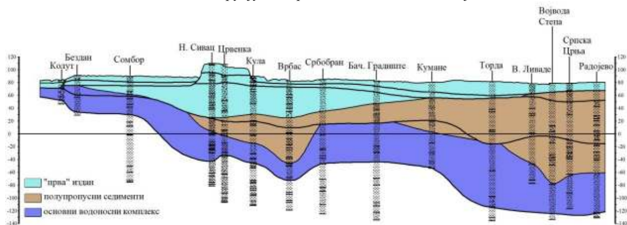
Слика 6: Хидрогеолошки пресек на подручју Бачке и Баната (правац запад-исток)
