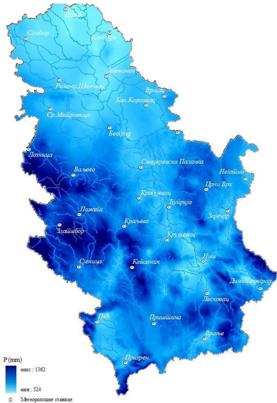
Слика 2: Просечне вишегодишње суме падавина
