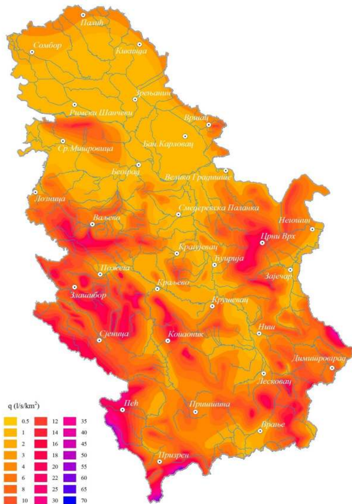
Слика 3: Модули отицаја
